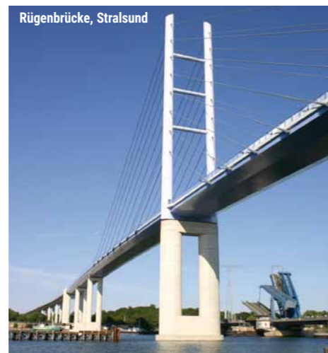
Rügenbrücke, Stralsund
